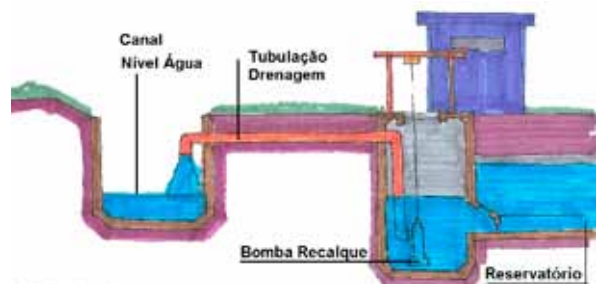
Figura 5. Funcionamento de um piscinão, tipo “Off-Line”. Fonte: DAEE, 2016, ilustração do autor.
