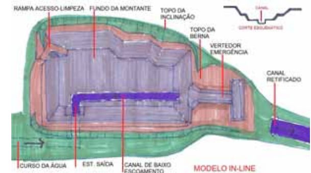
Figura 4. Piscião - IN-LINE. Fonte: DAEE, 2016, ilustração do autor.
